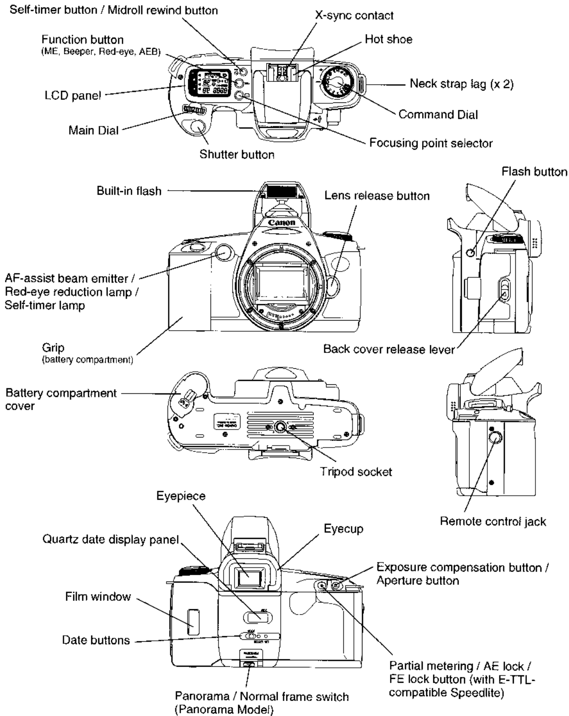
Fig. 1-10 Nomenclature
