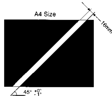
Fig. 3-6 45° Bar Chart
