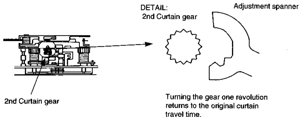
Fig. 3-63 Shutter Spanner
