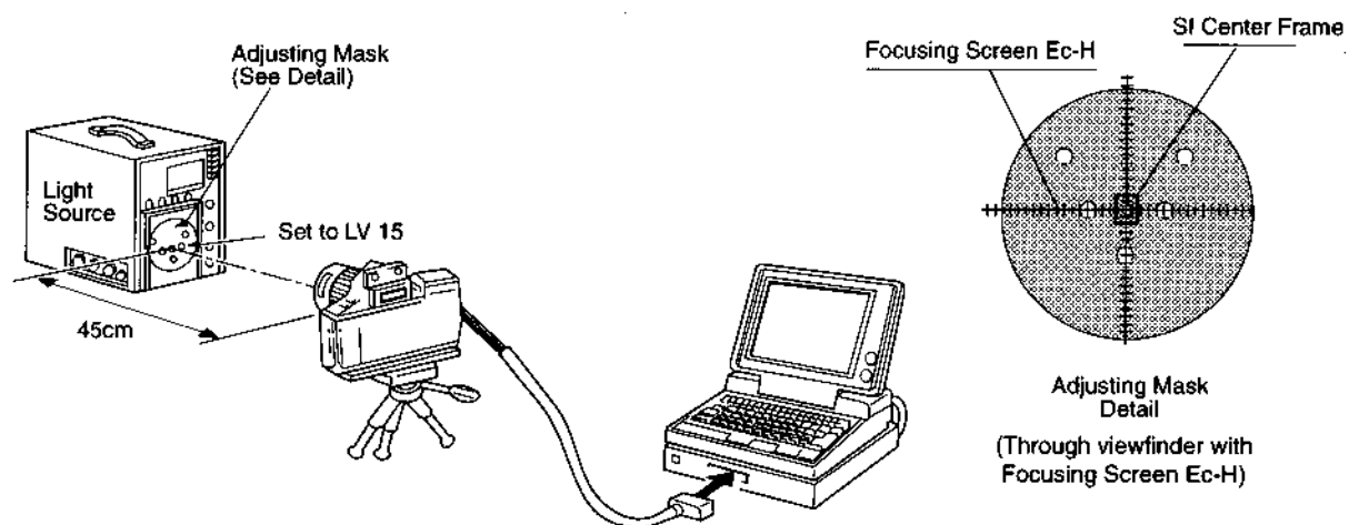
Fig. 3-89 SPD Positioning
